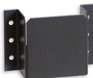
Art.940-06 Supporto da parete per FA-07 Dimensioni: 11,5x8x4,2cm. - Peso: 0,2kg.
