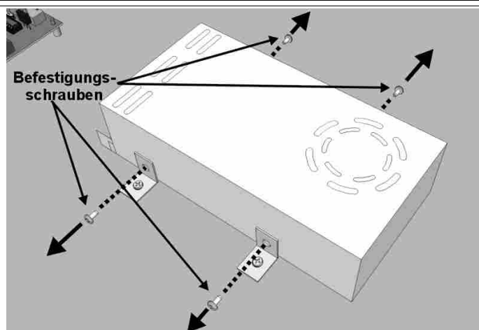
Fig. 22: Ersetzen des Netzteils
