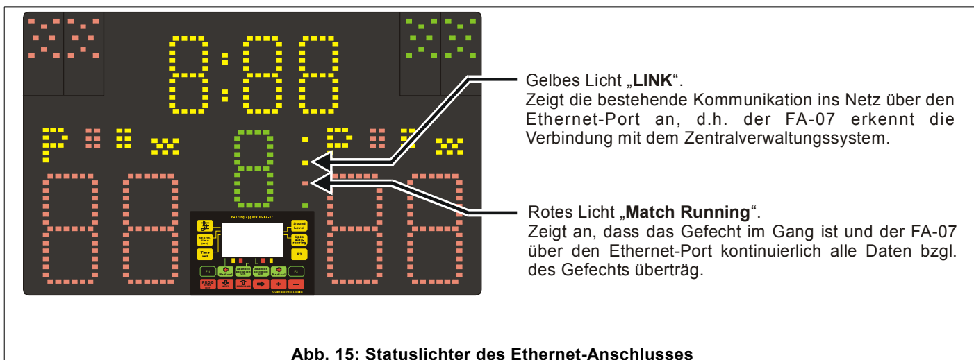
Abb. 15: Statuslichter des Ethernet-Anschlusses
