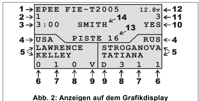
Abb. 2: Anzeigen auf dem Grafikdisplay
